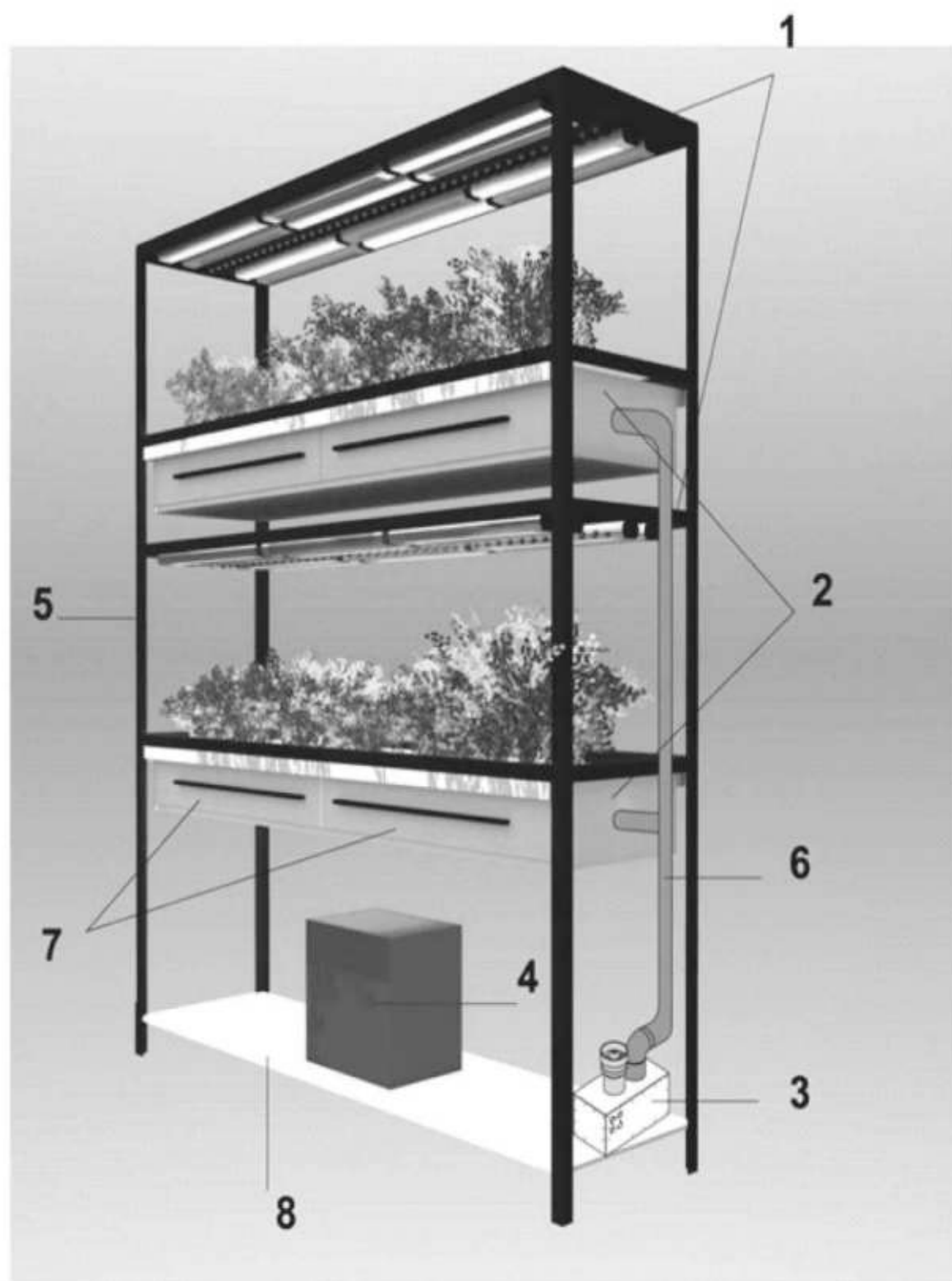
Рис. 2. Внешний вид биотехнологической установки:
